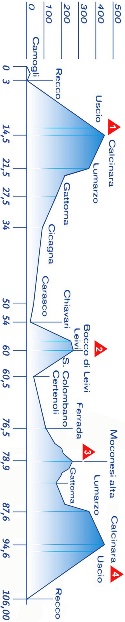
PROFILO ALTIMETRICO _ distanza Km. 106,00 _ dislivello 1650 mt
